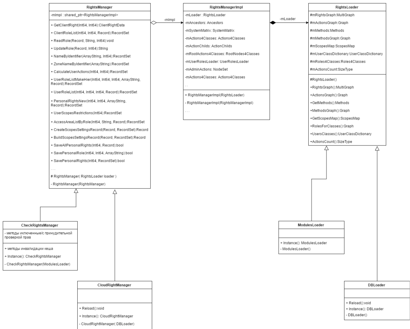
Рис. 1. Схема классов и их взаимодействие
